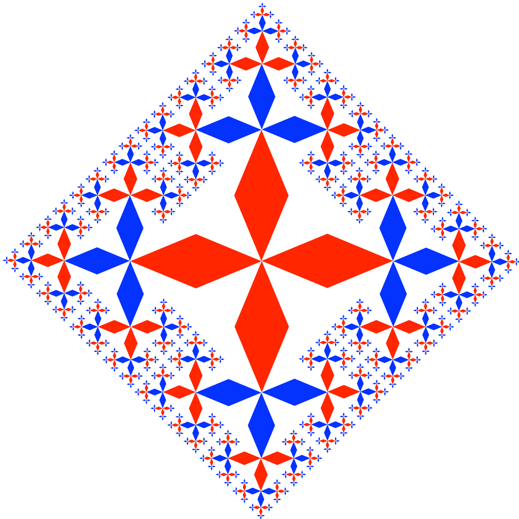
Abb. 4: Kreuze
