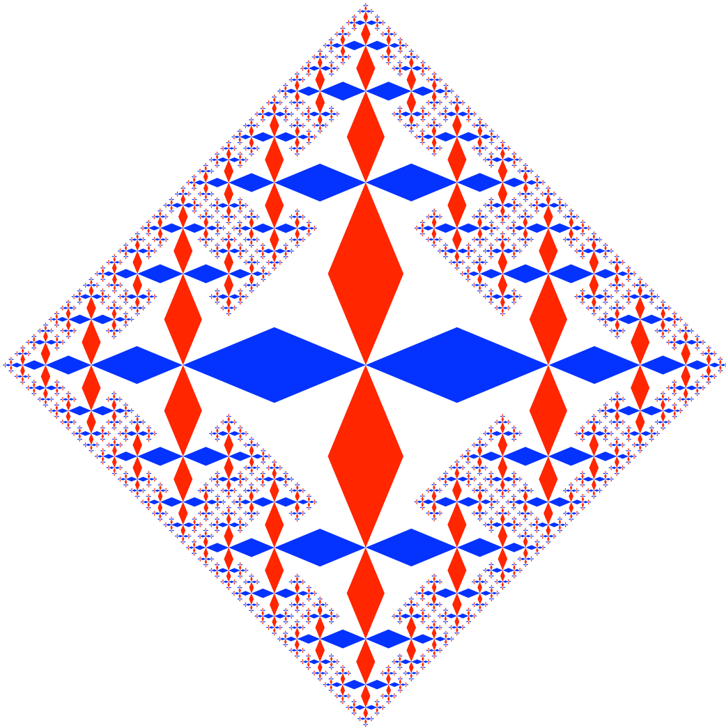
Abb. 5: Andere Färbung
