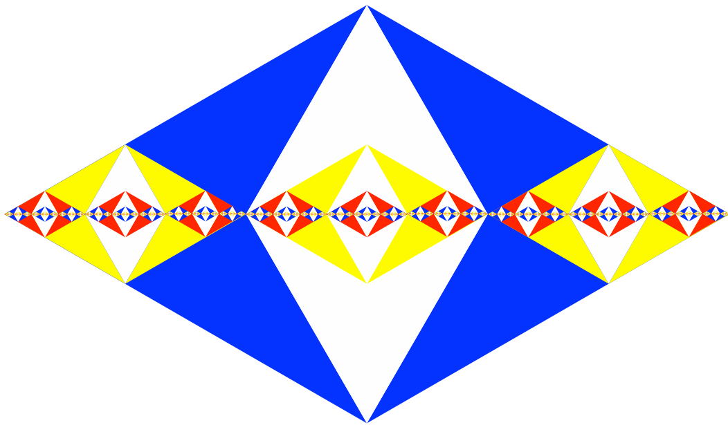
Abb. 2: Andere Färbung
