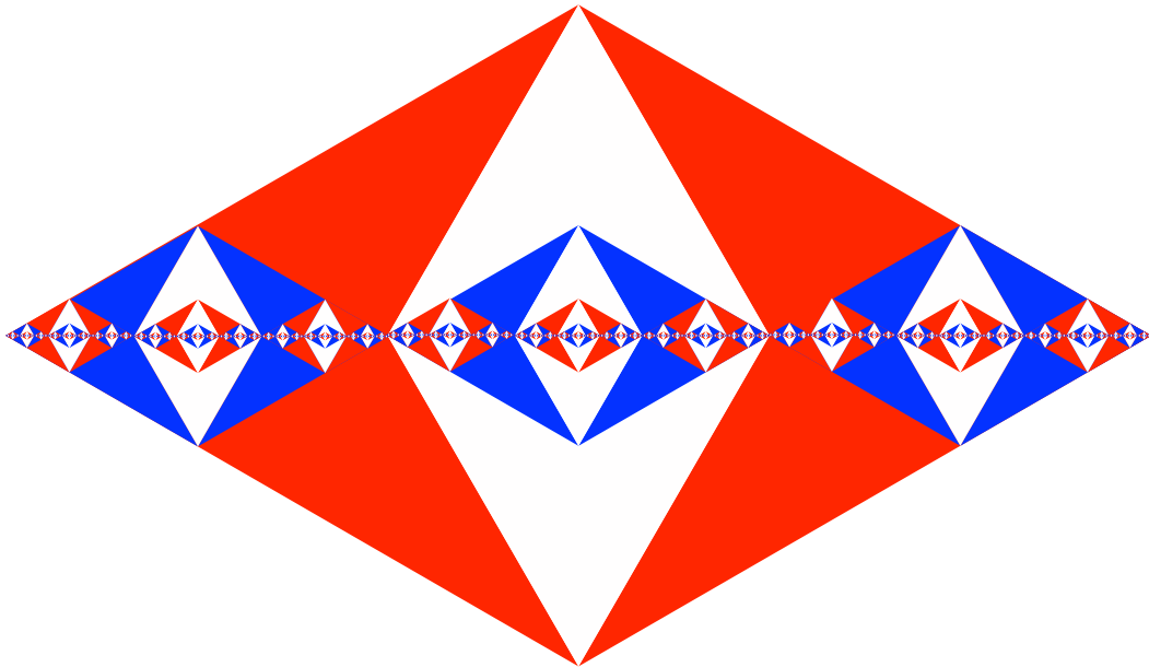
Abb. 1: 60°-Rhomben
