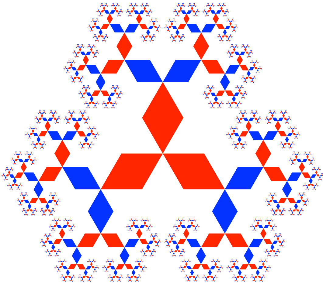
Abb. 3: Boabab
