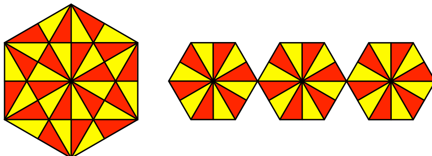
Abb. 3: Zerlegungsbeweis
