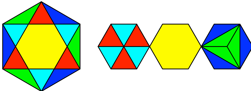
Abb.2: Zerlegungsbeweis
