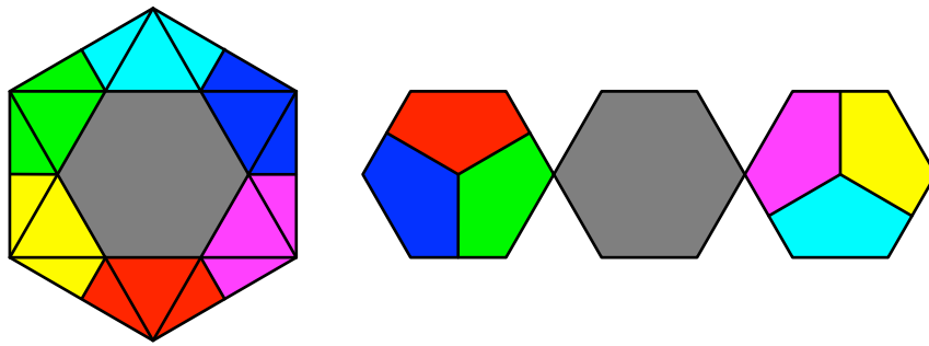
Abb. 4: Zerlegungsbeweis
