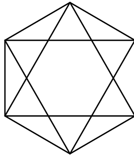
Abb. 1: Sechsecke
