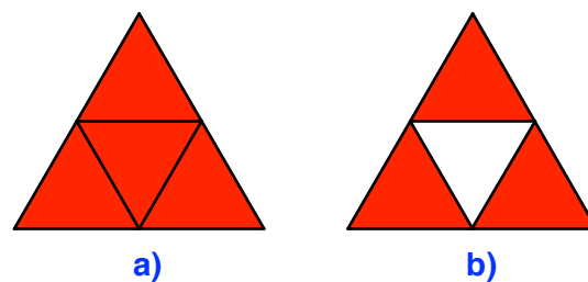
Abb. 1: Sierpinksi-Dreieck
