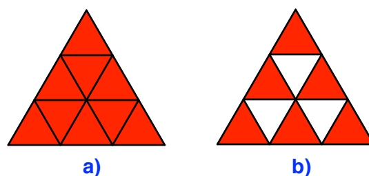
Abb. 2: Variante
