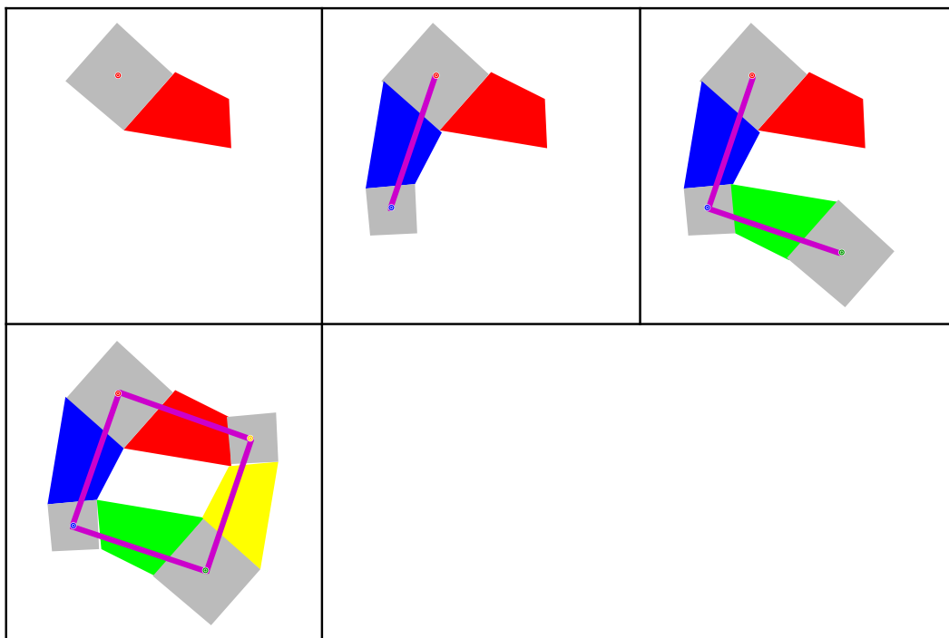
Kongruente Vierecke und Quadrate
