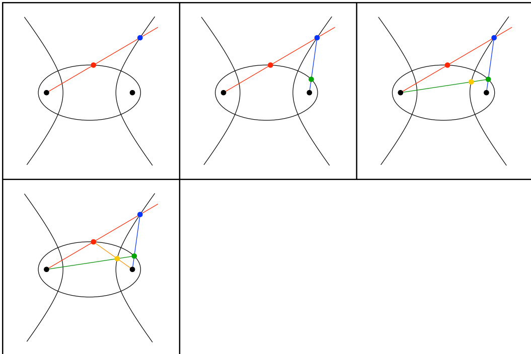
Ellipse und Hyperbel mit gemeinsamen Brennpunkten
