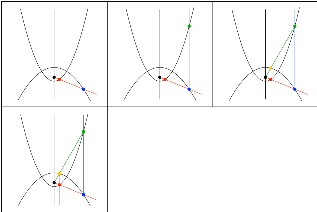
Konfokale Parabeln
