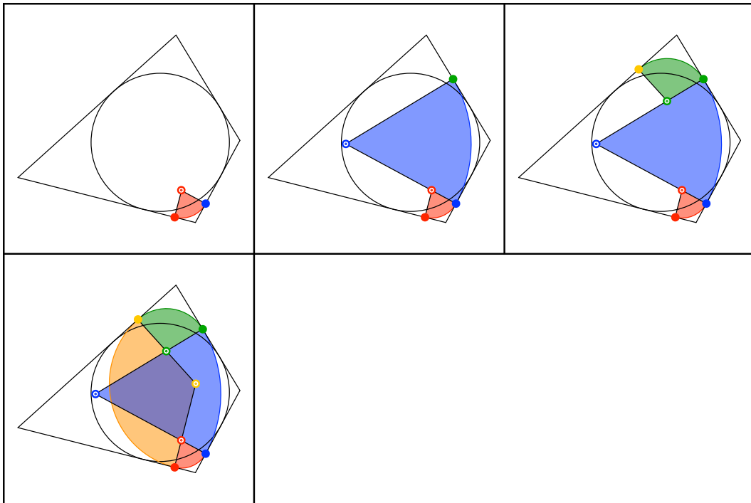
Tangentenviereck
