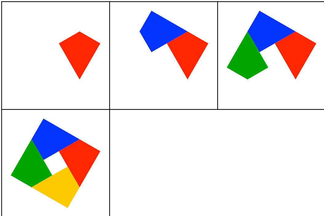
Drachen mit rechten Winkeln
