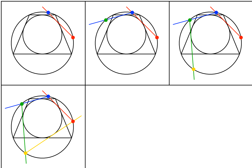
Sehnen-Tangentenviereck
