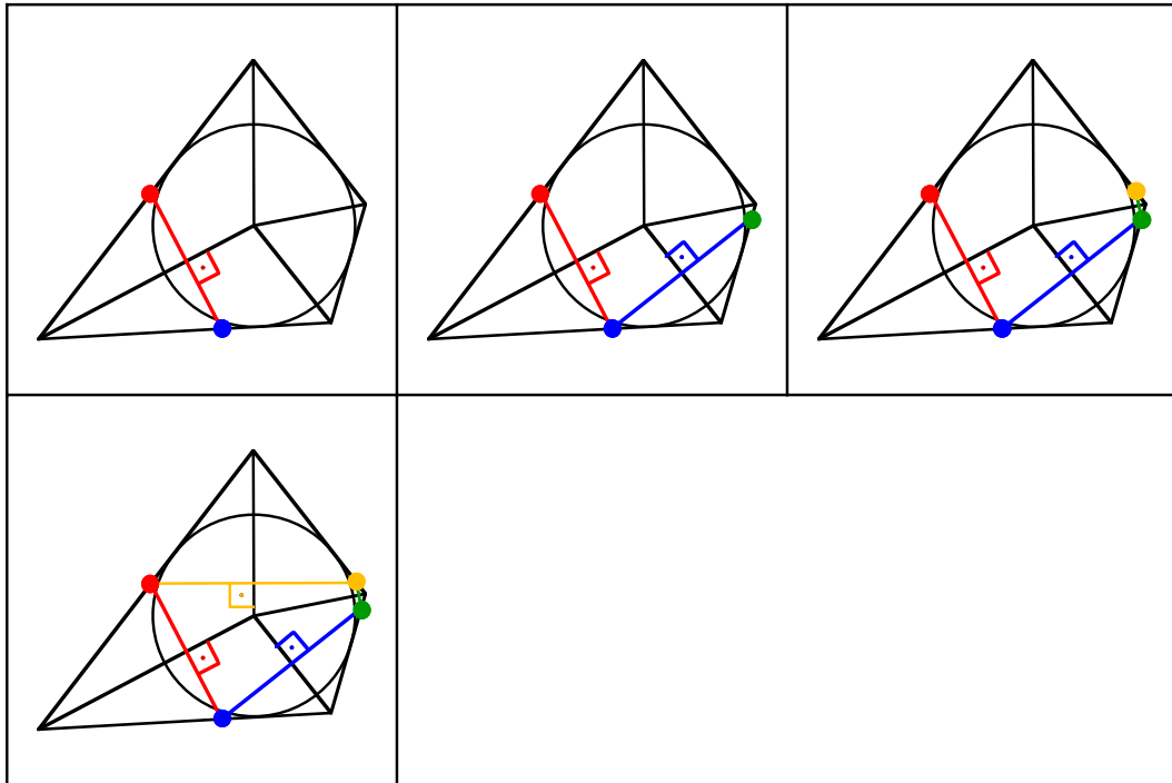
Tangentenviereck
