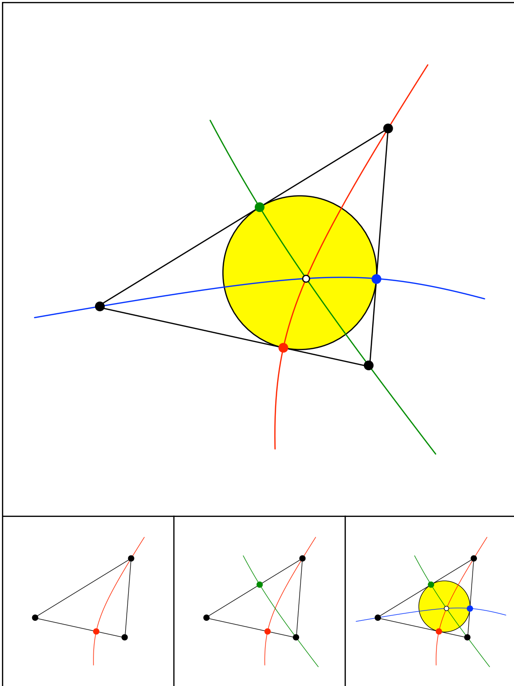
Hyperbeln
