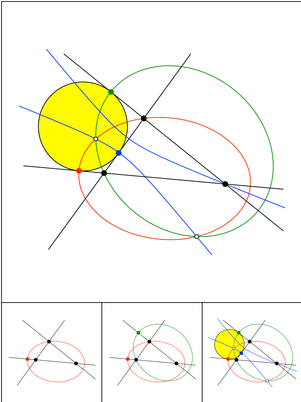
Zwei Ellipsen und eine Hyperbel
